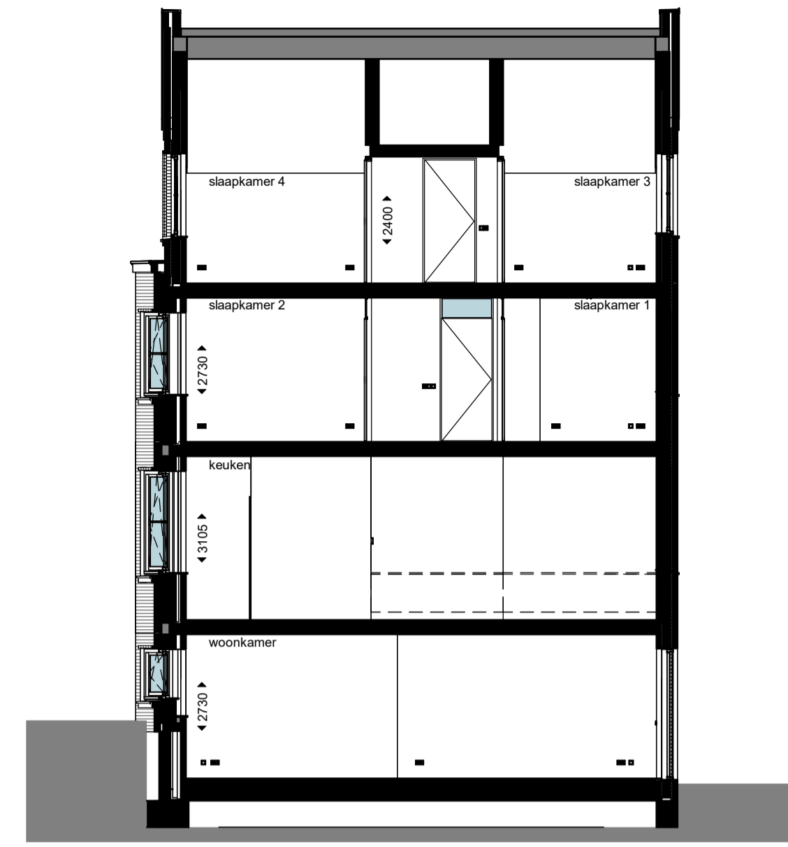
doorsnede
