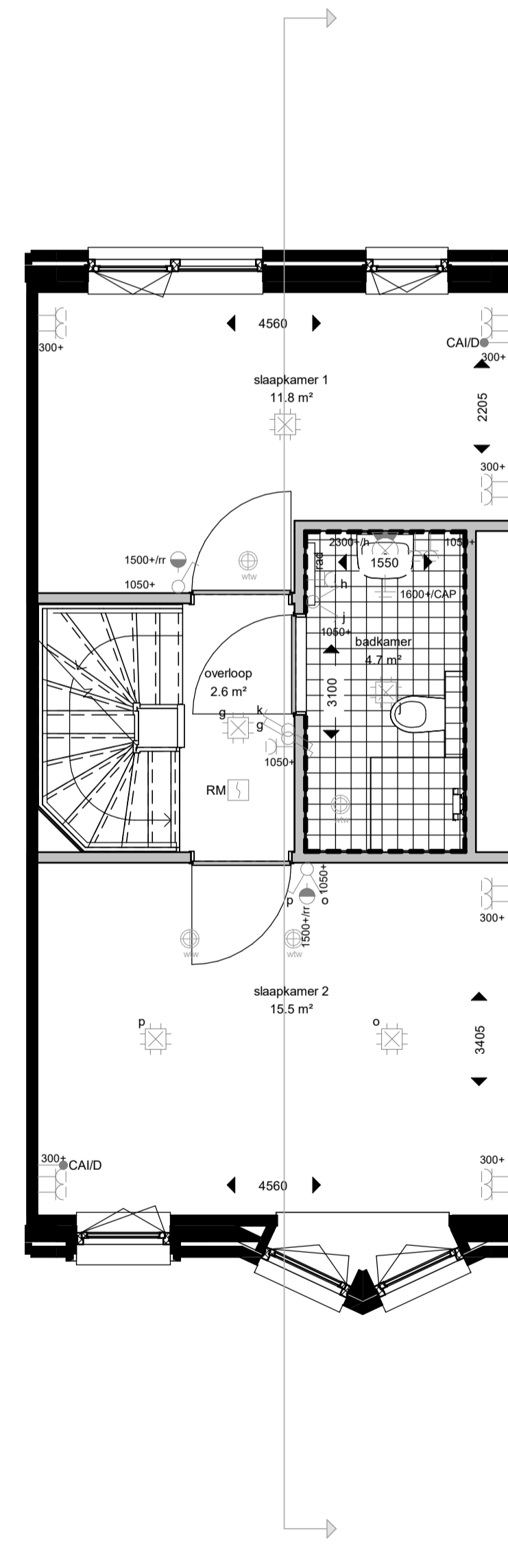
eerste verdieping
