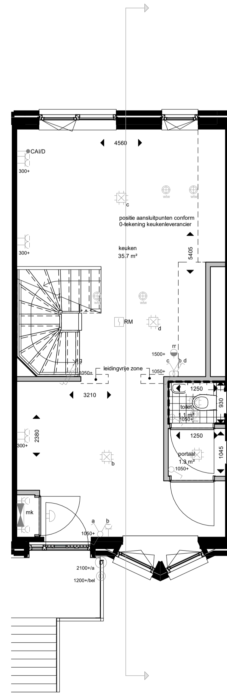
beletage
