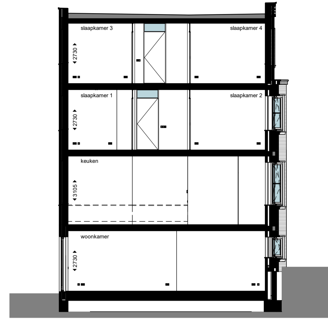
doorsnede
