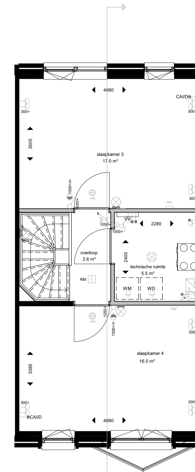
tweede verdieping
