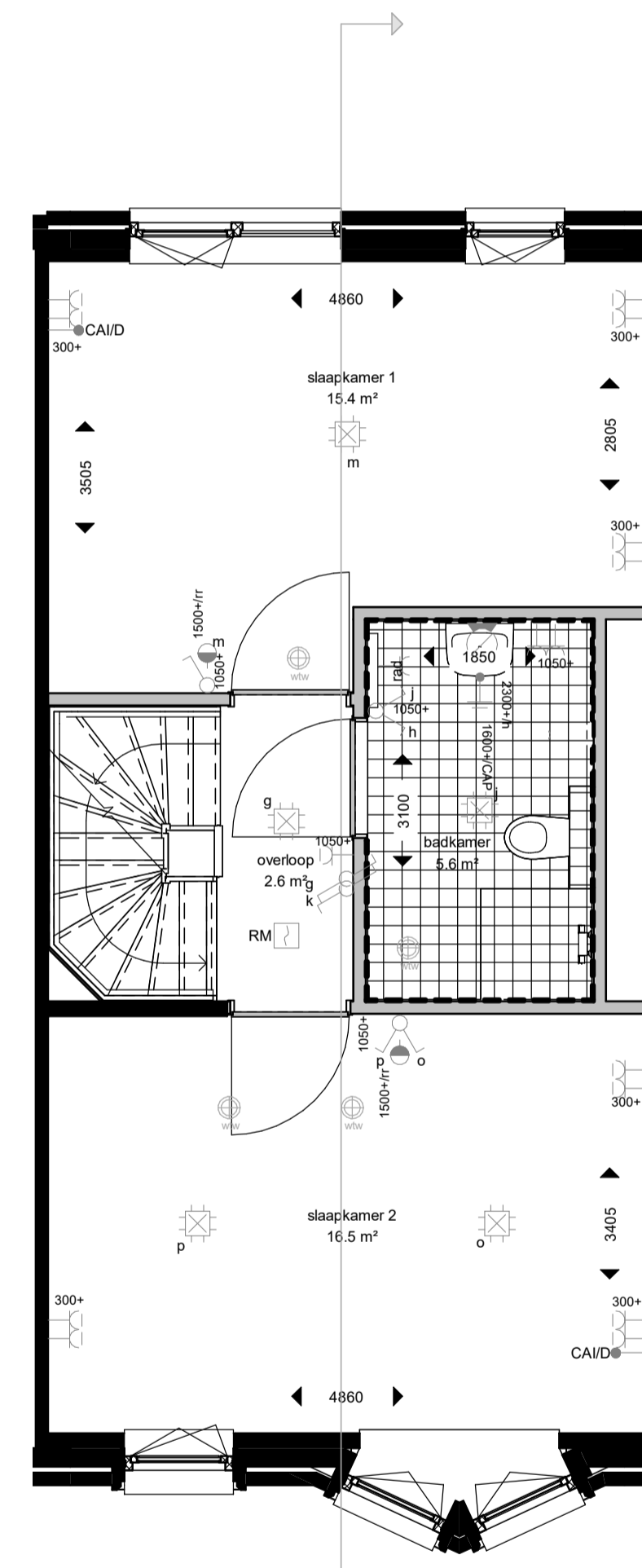
eerste verdieping
