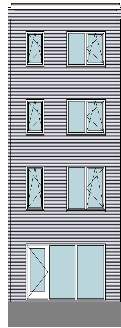
achtergevel
