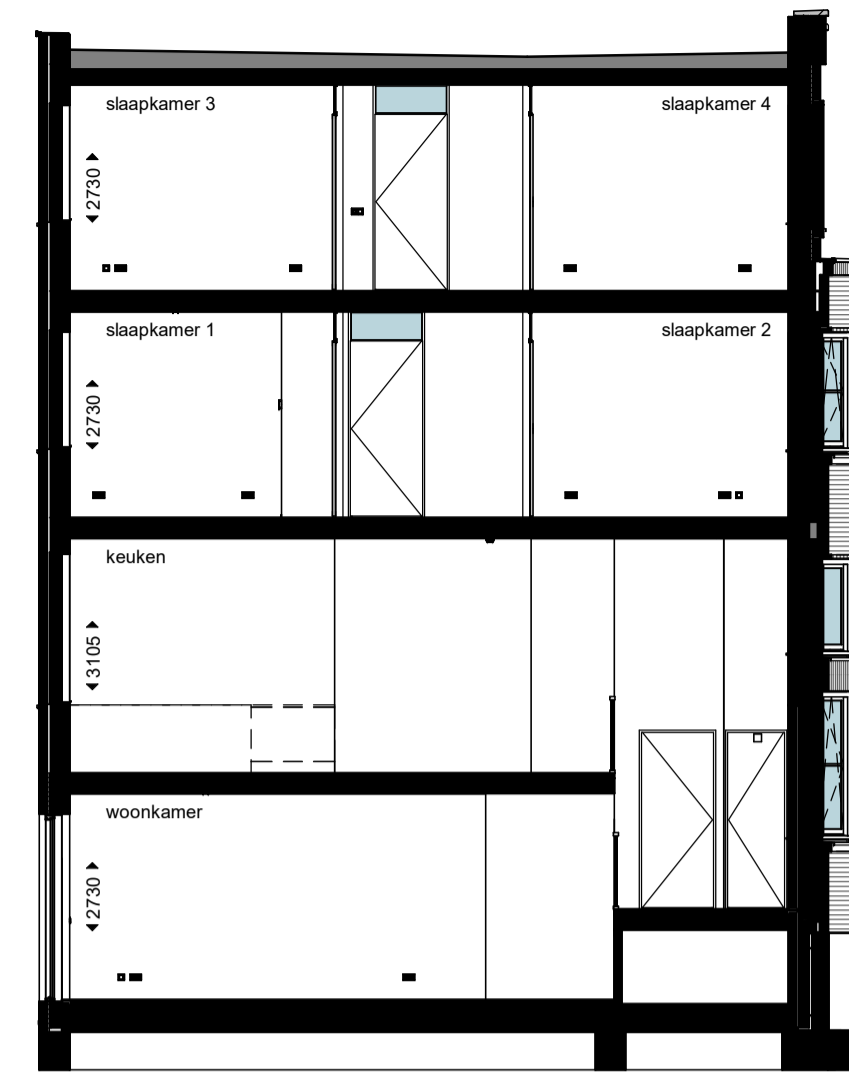
doorsnede
