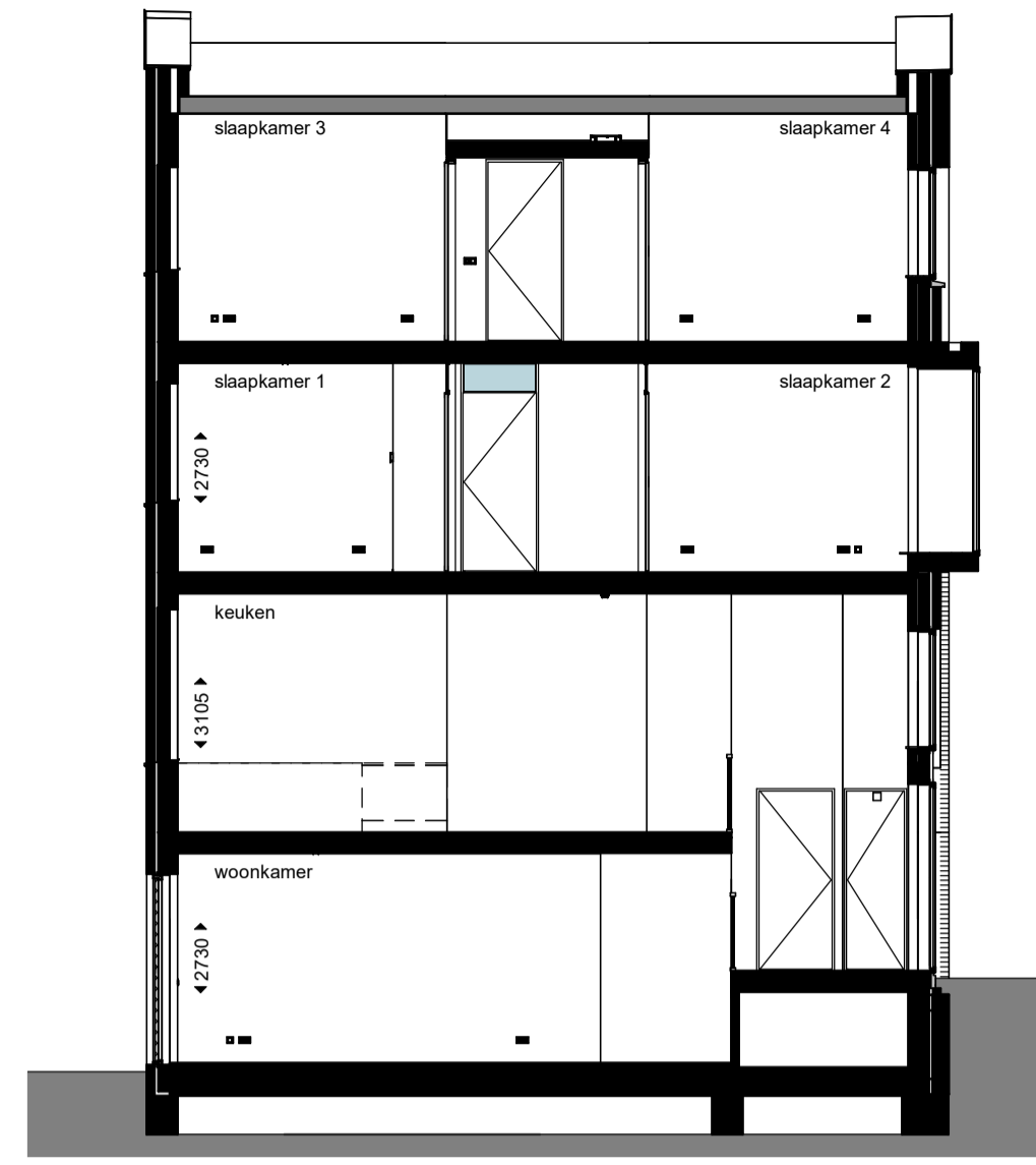
doorsnede
