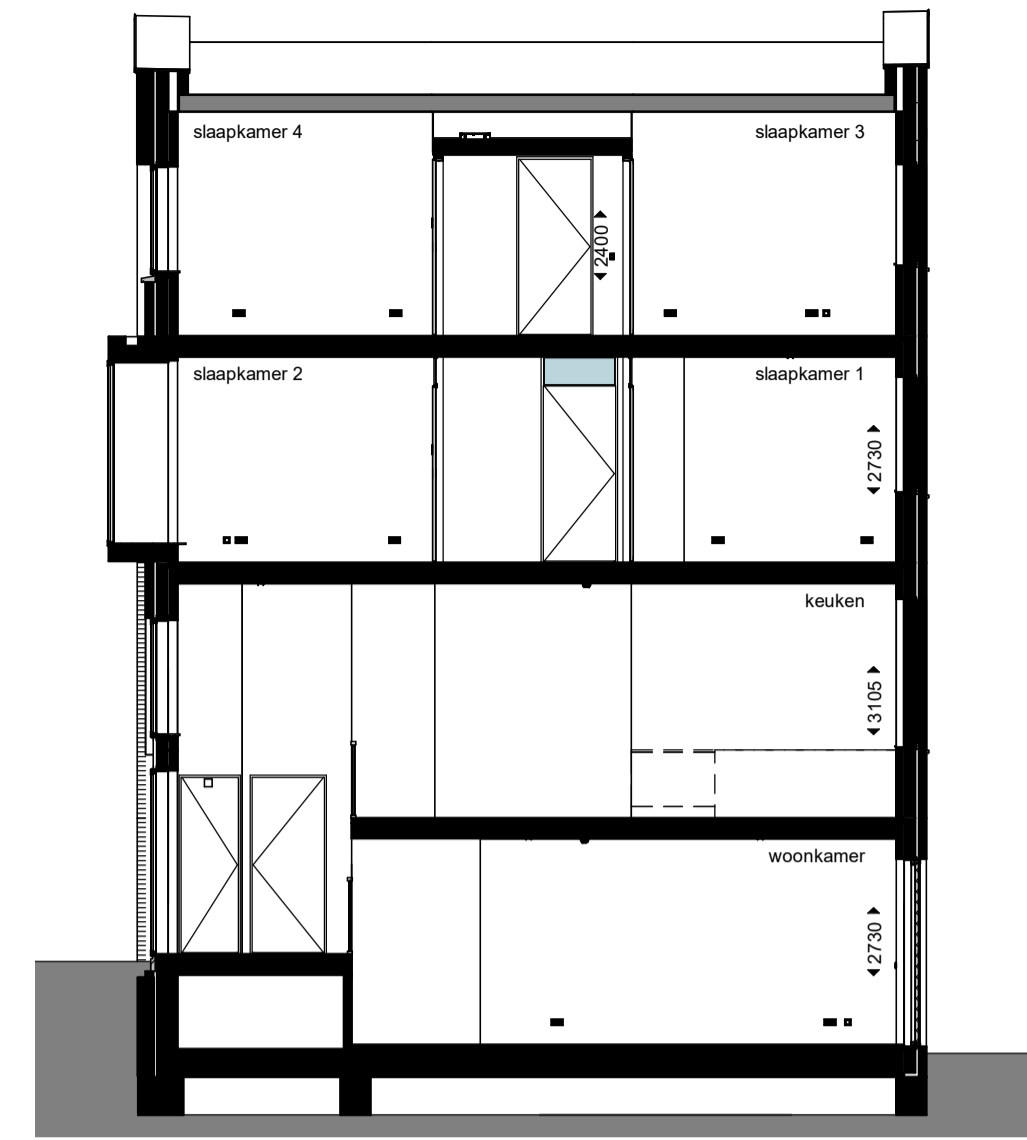
doorsnede
