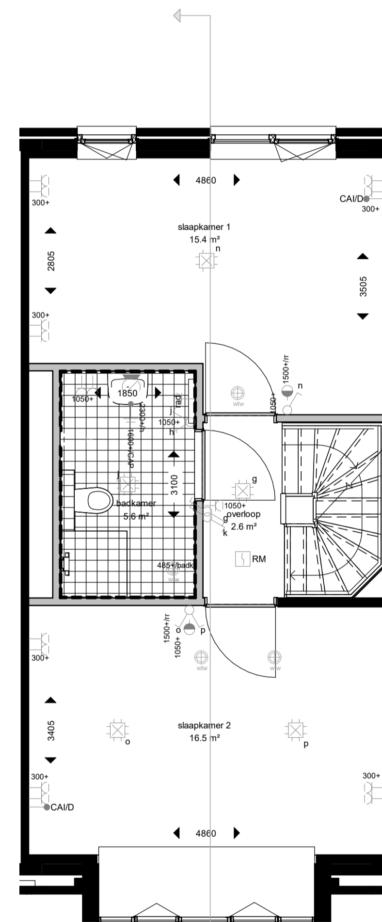
eerste verdieping
