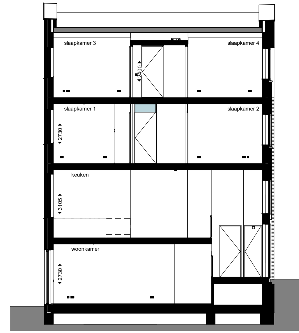
doorsnede
