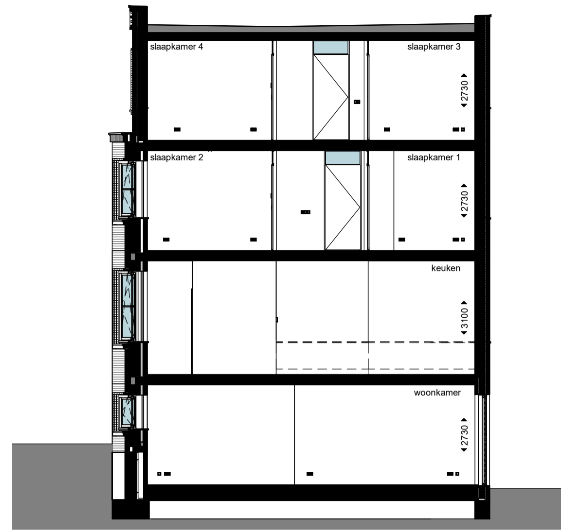
doorsnede
