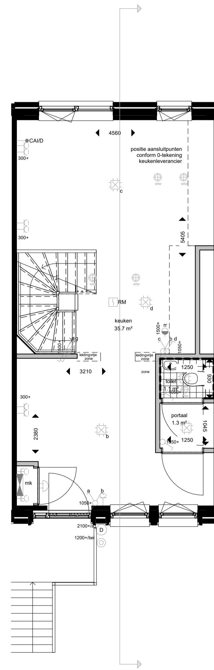
beletage
