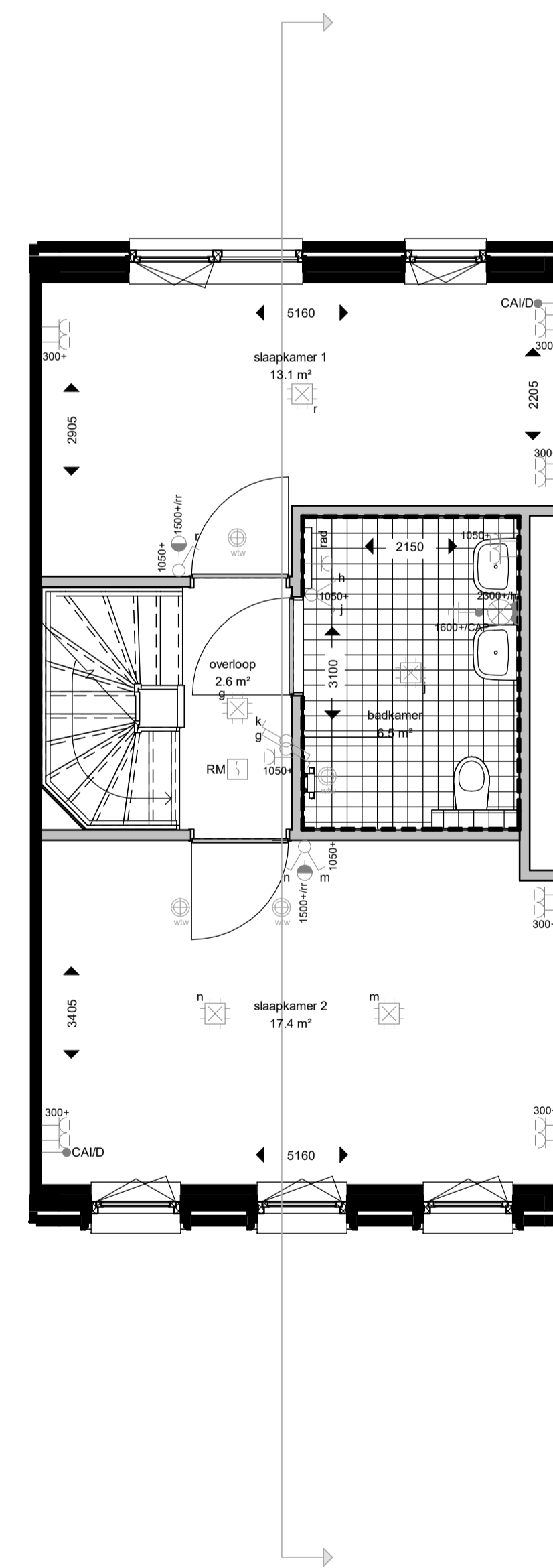
eerste verdieping
