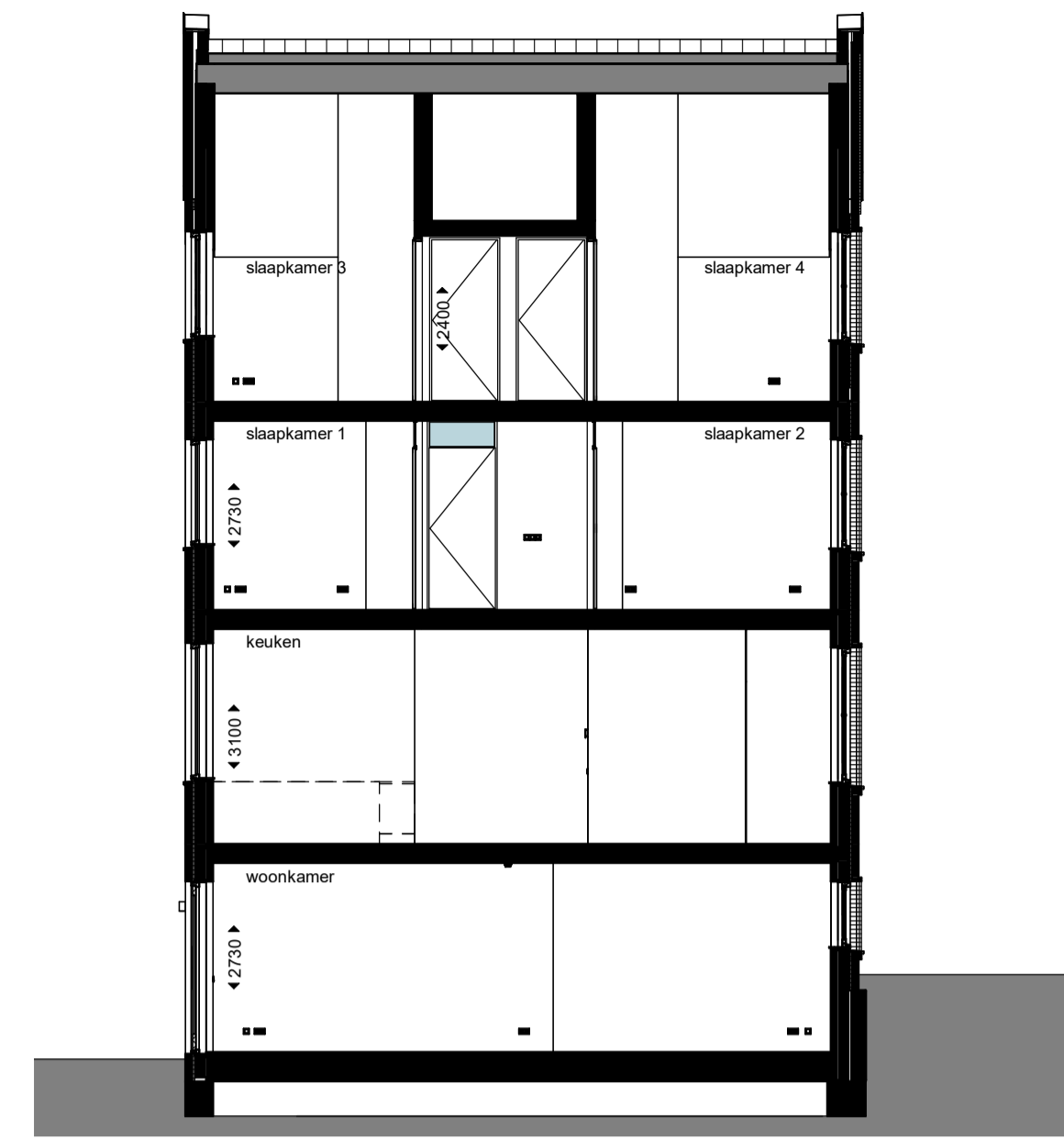
doorsnede
