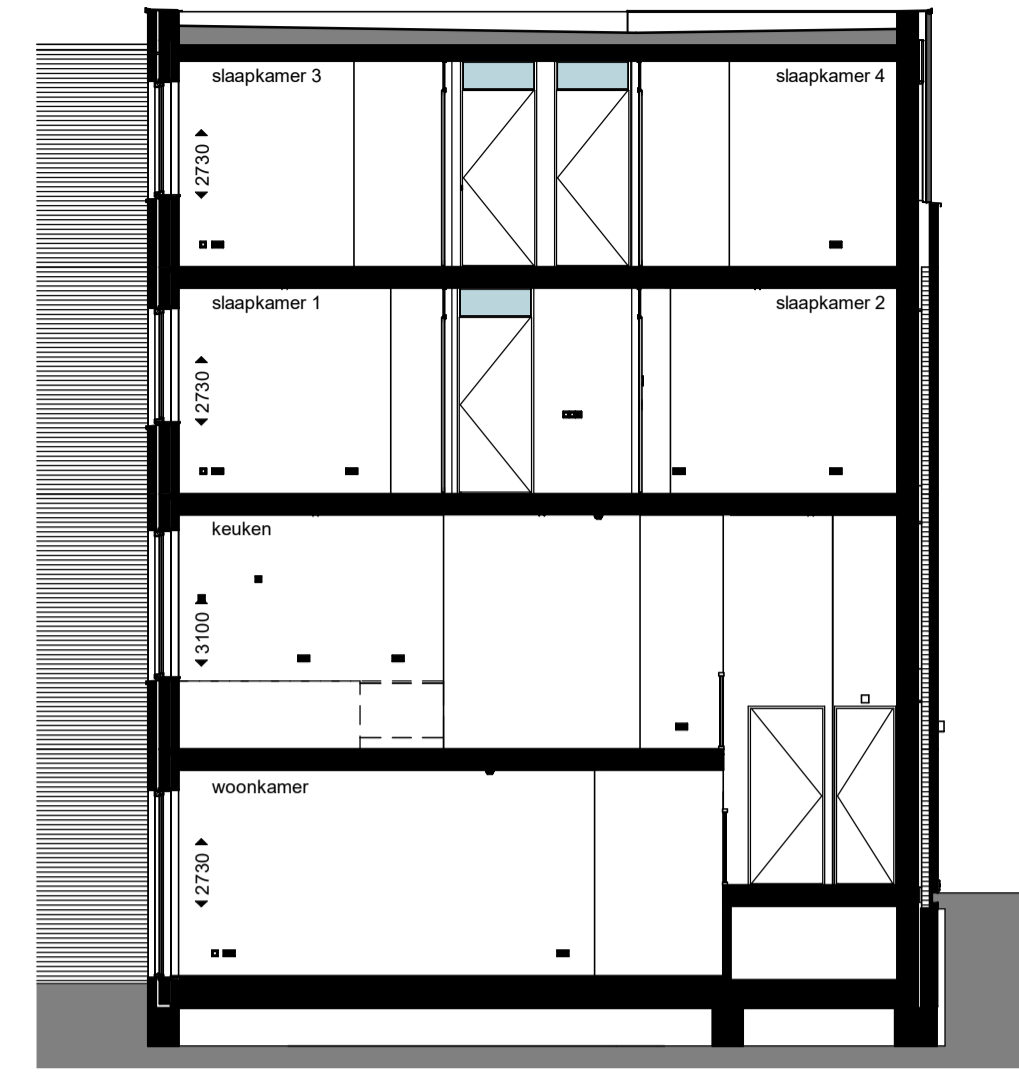
doorsnede
