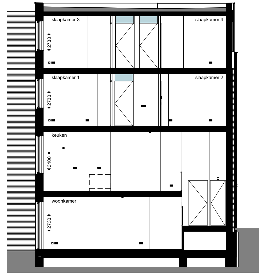
doorsnede
