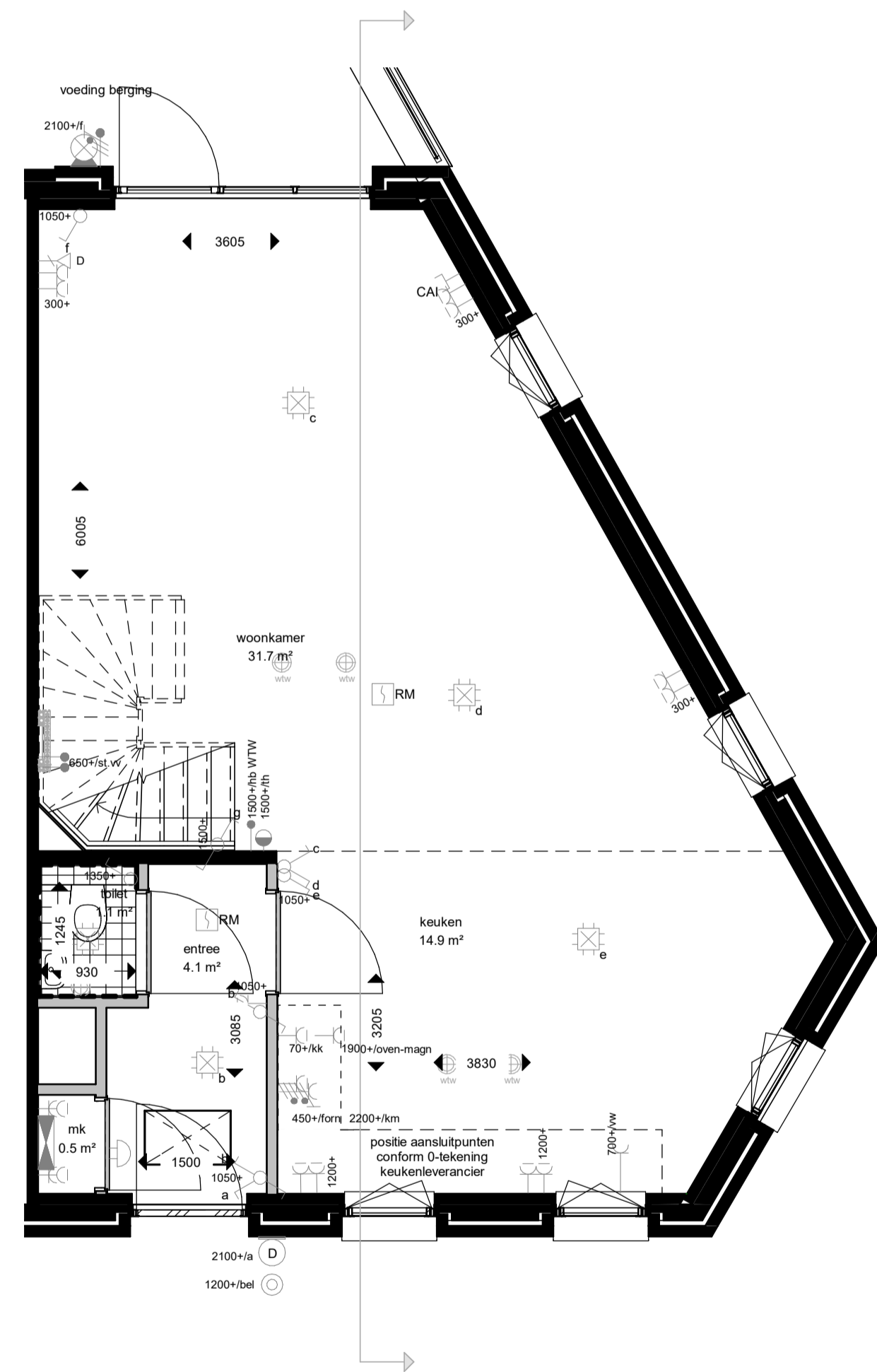
begane grond
