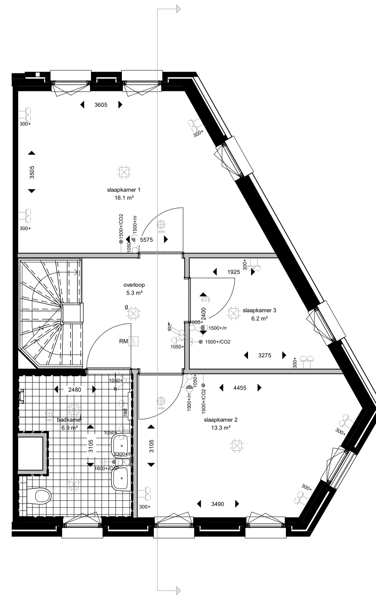
eerste verdieping
