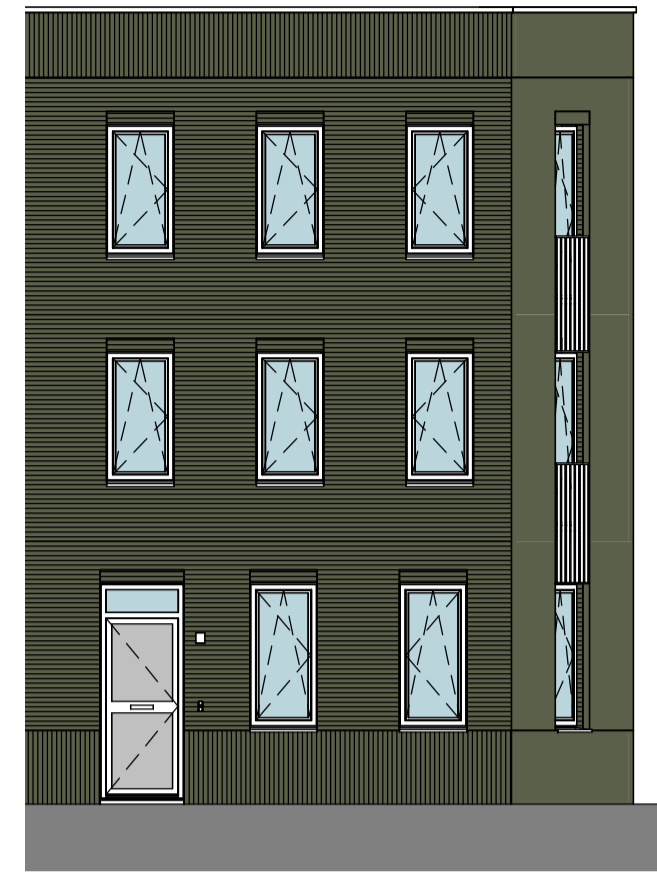
voorgevel
