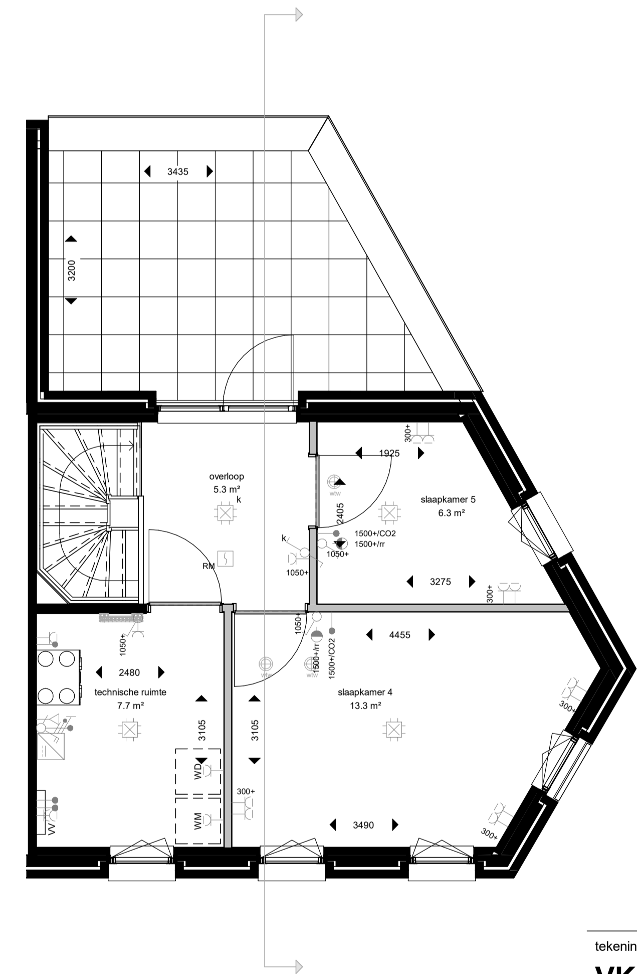
tweede verdieping
