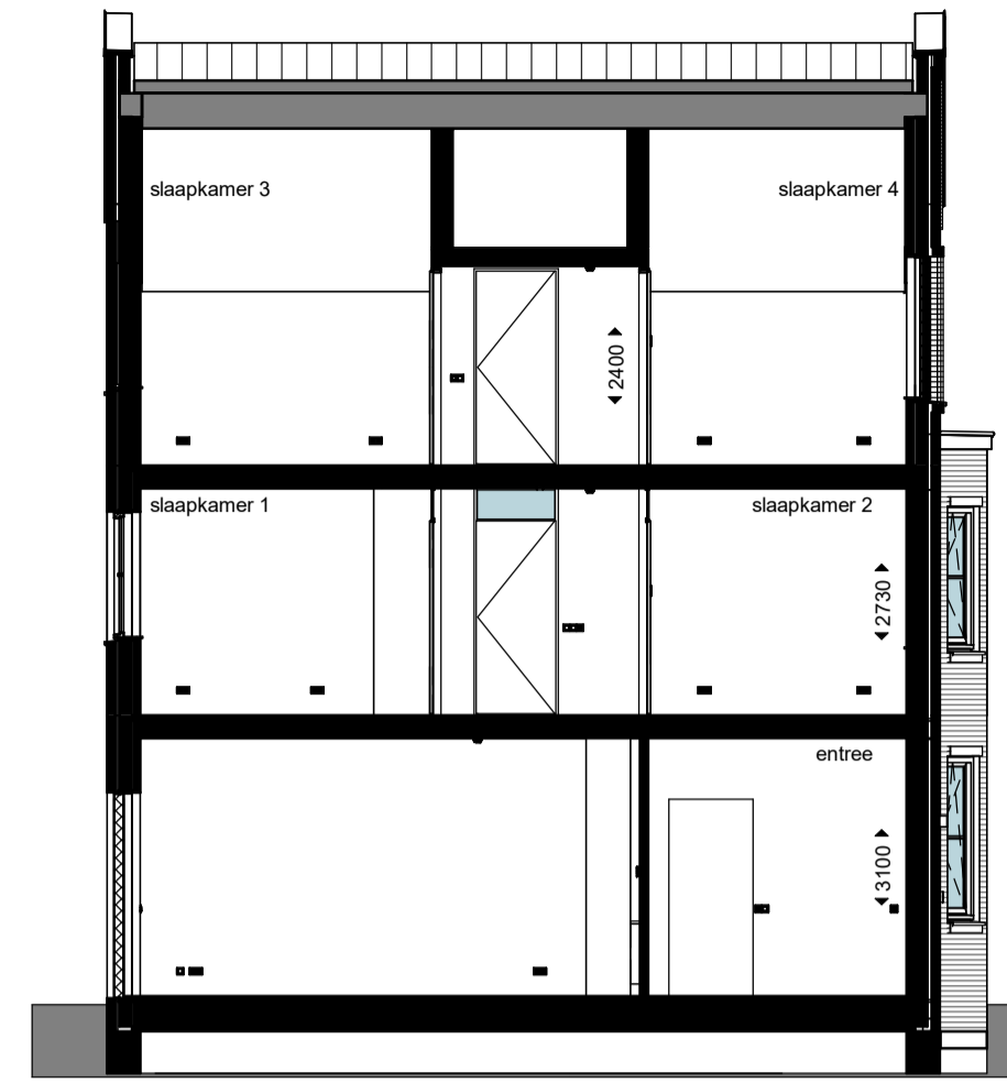
doorsnede
