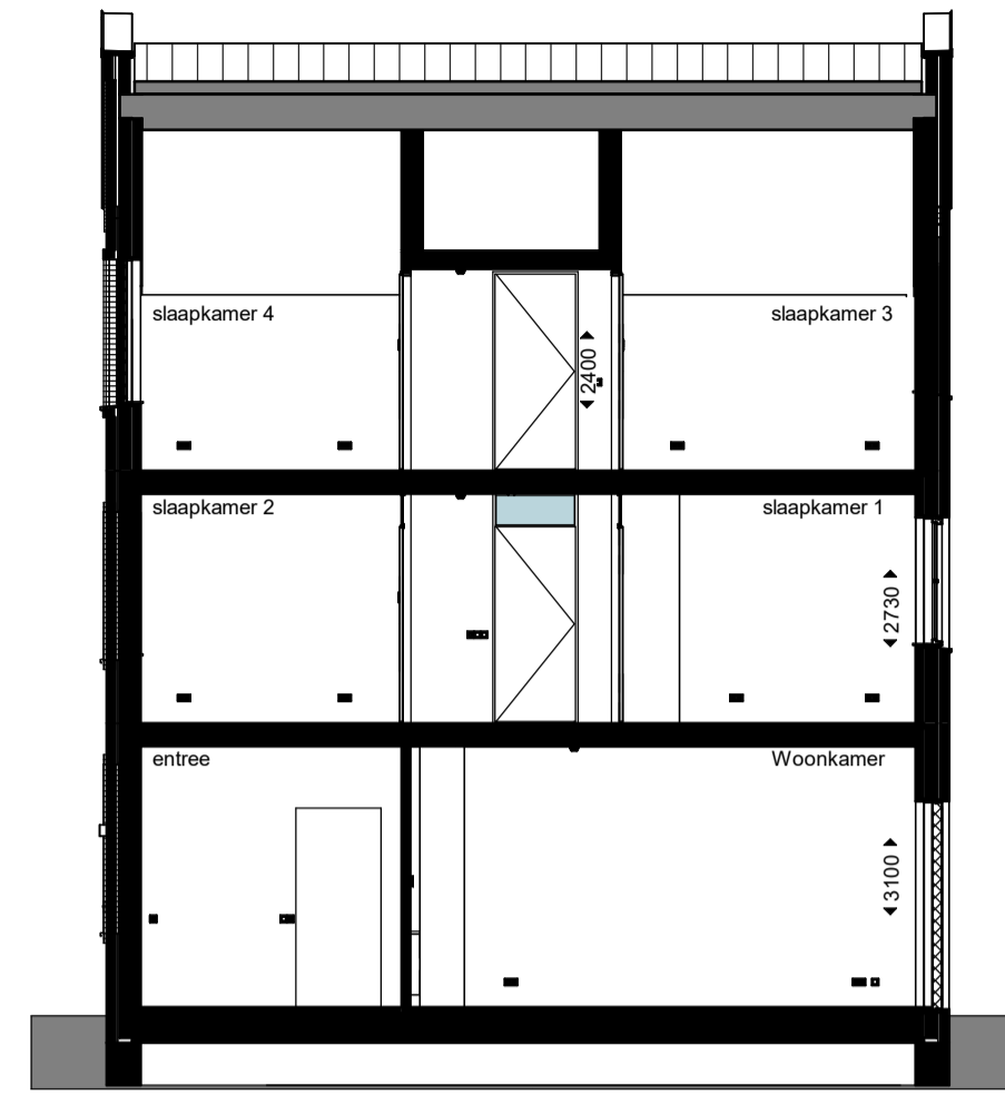
doorsnede
