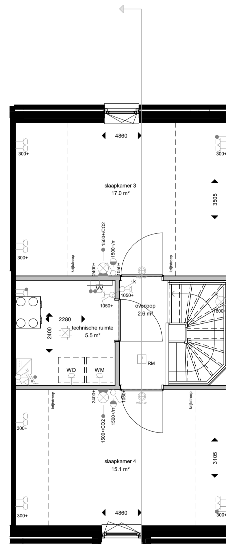
tweede verdieping
