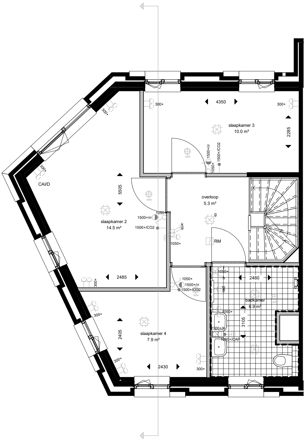
eerste verdieping
