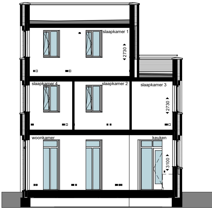
doorsnede
