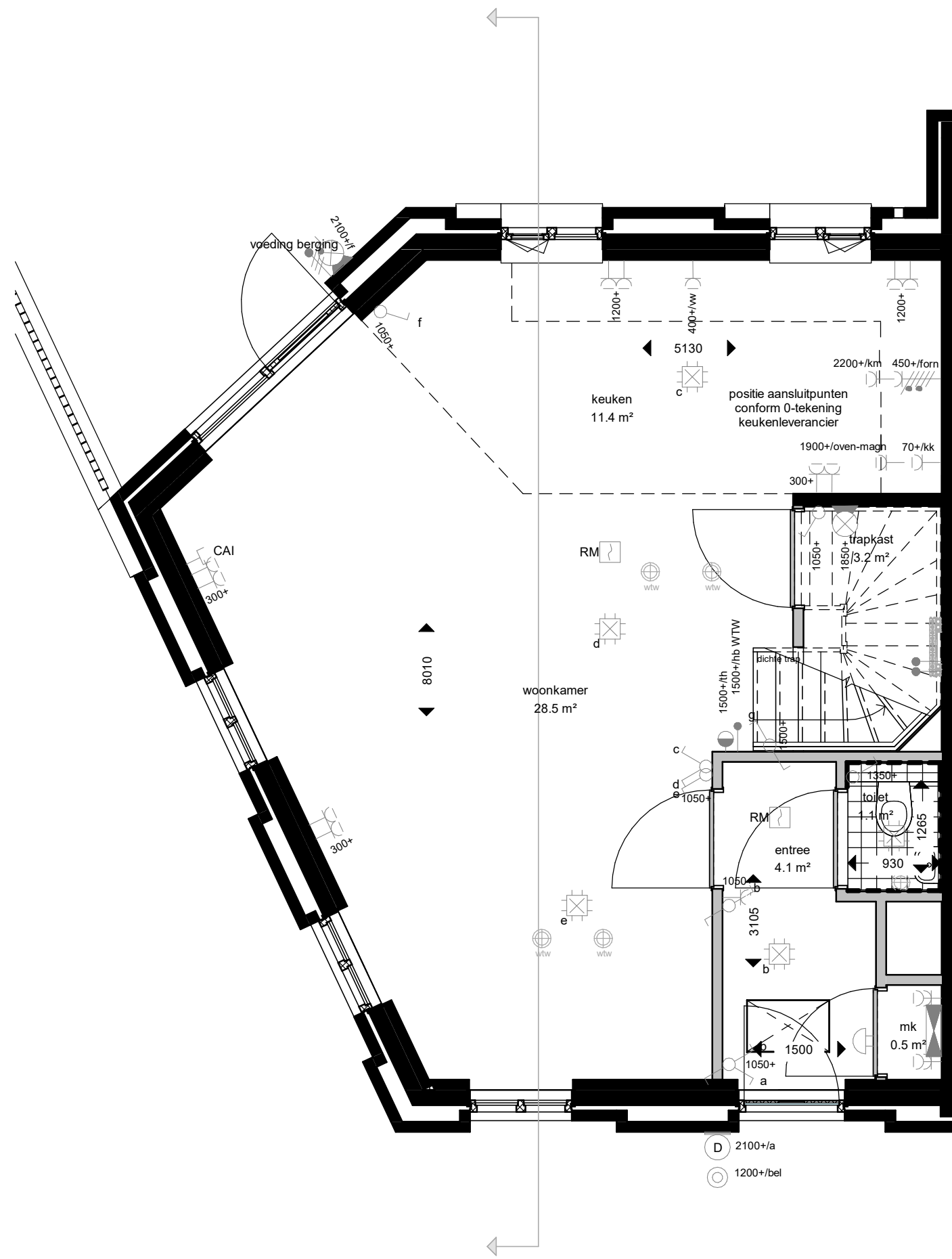
begane grond
