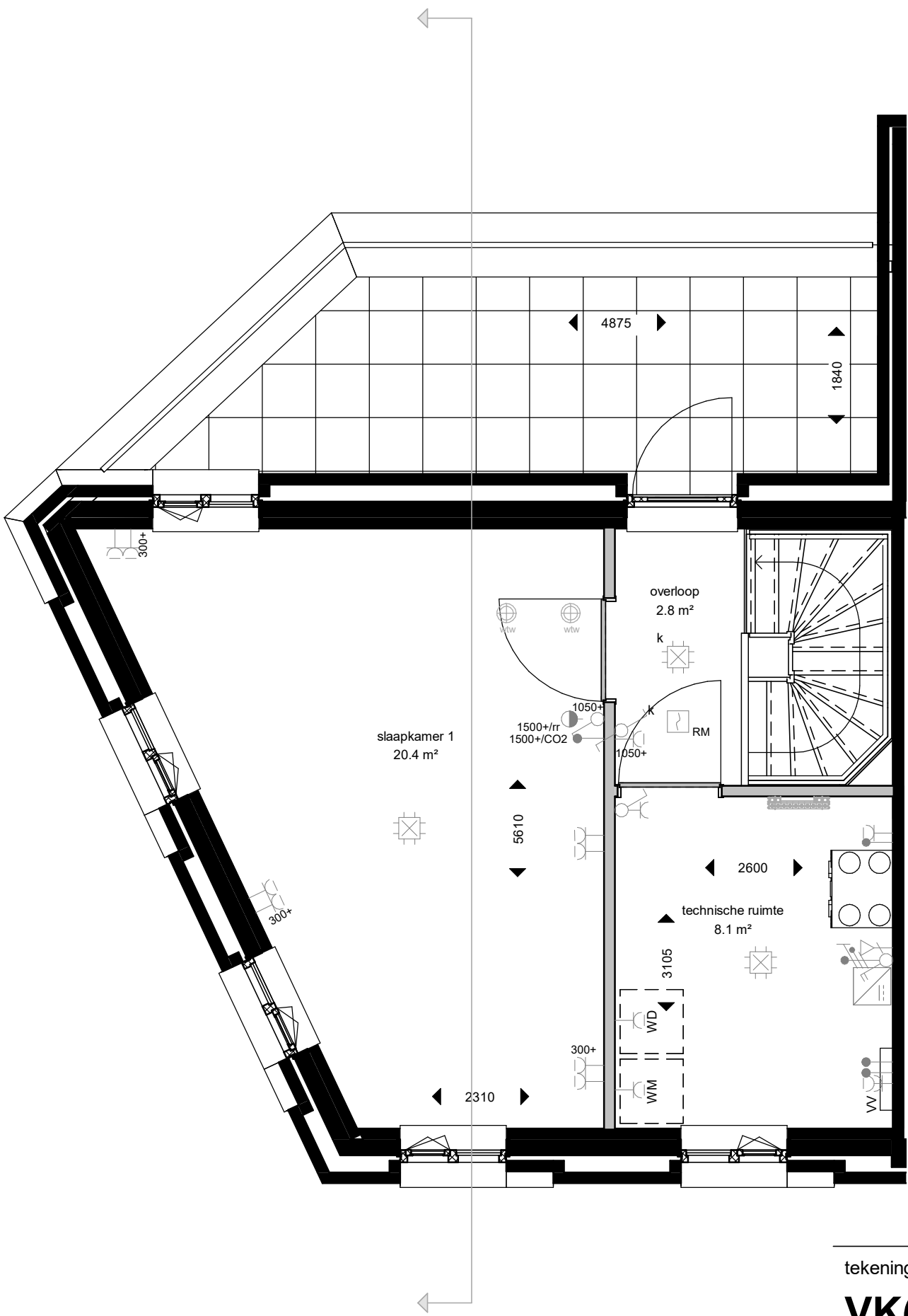
tweede verdieping
