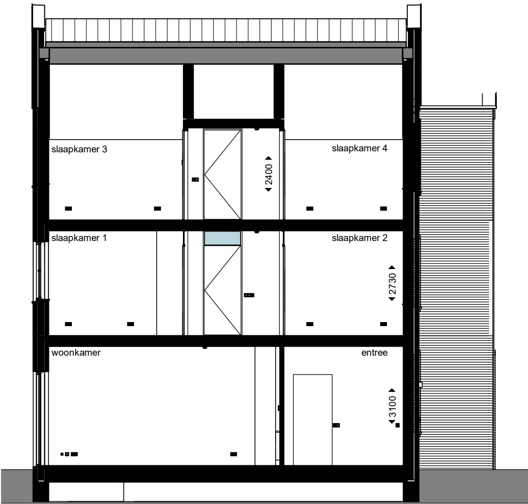
doorsnede
