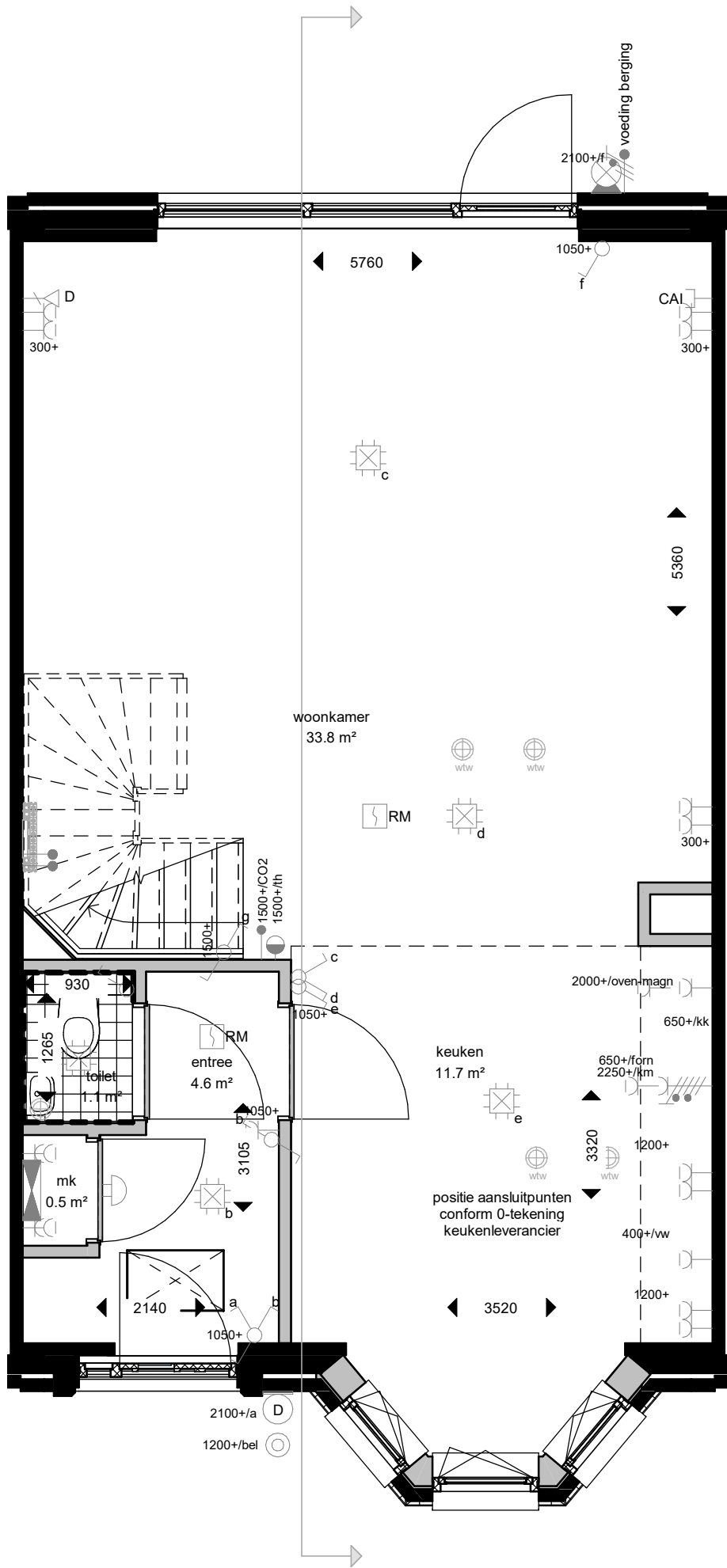
begane grond
