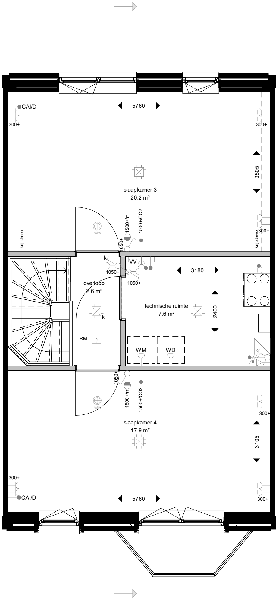
tweede verdieping
