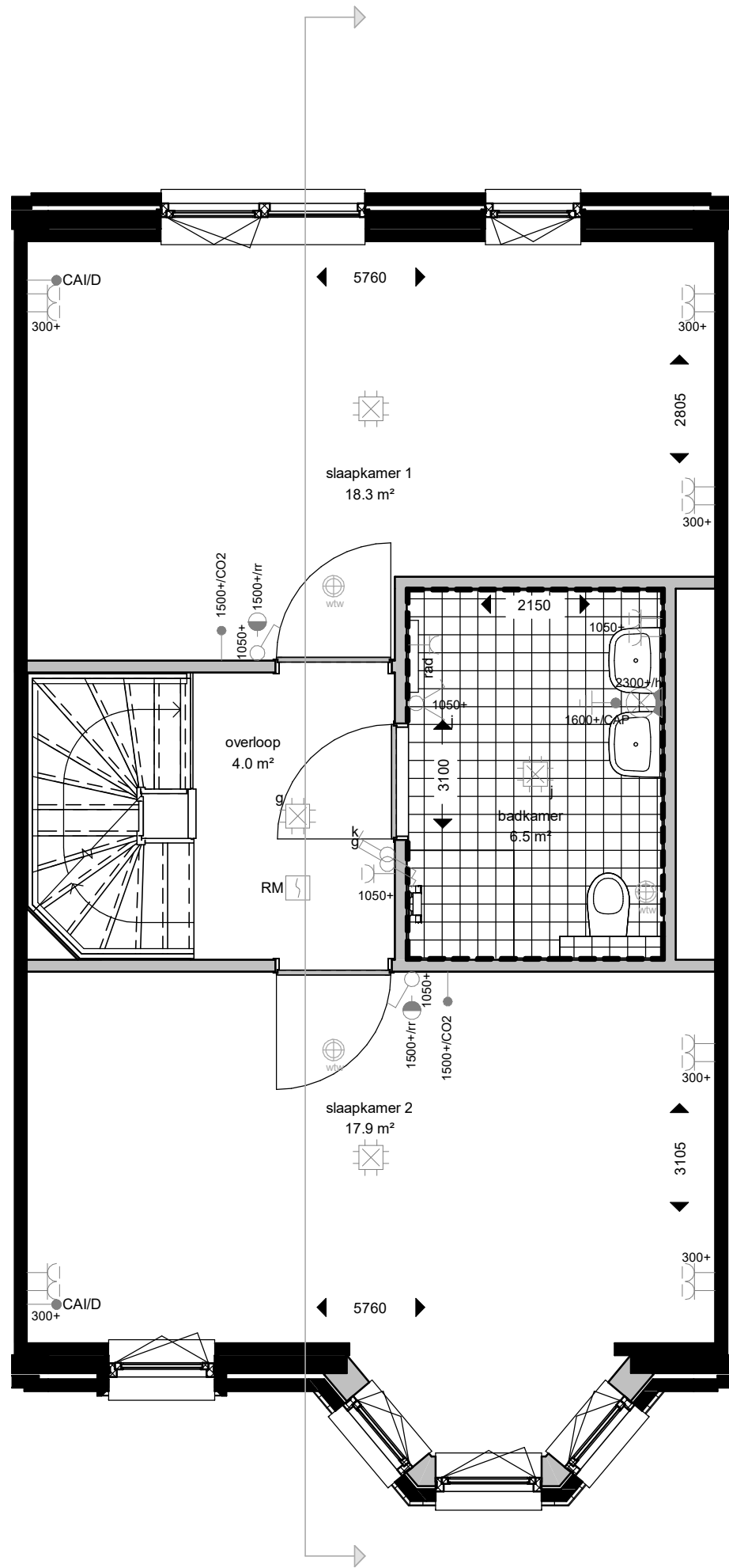
eerste verdieping
