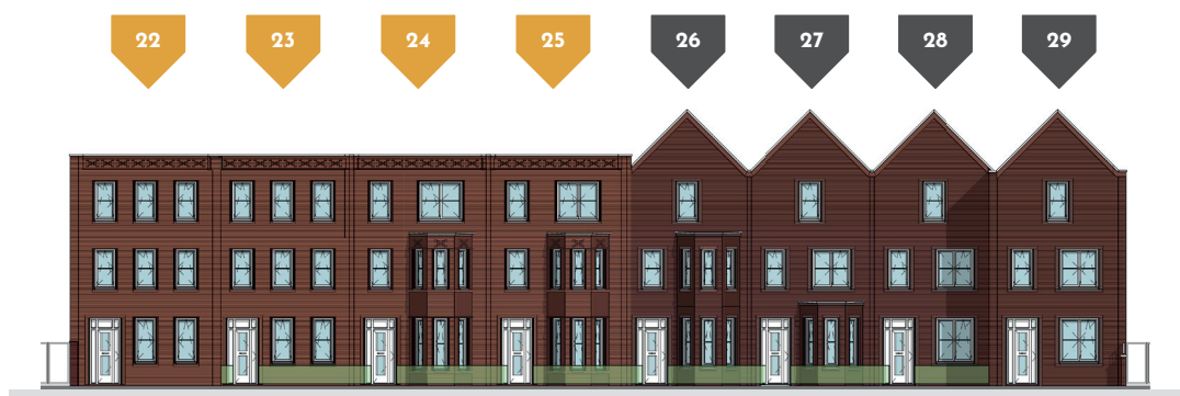
Voorgevel
