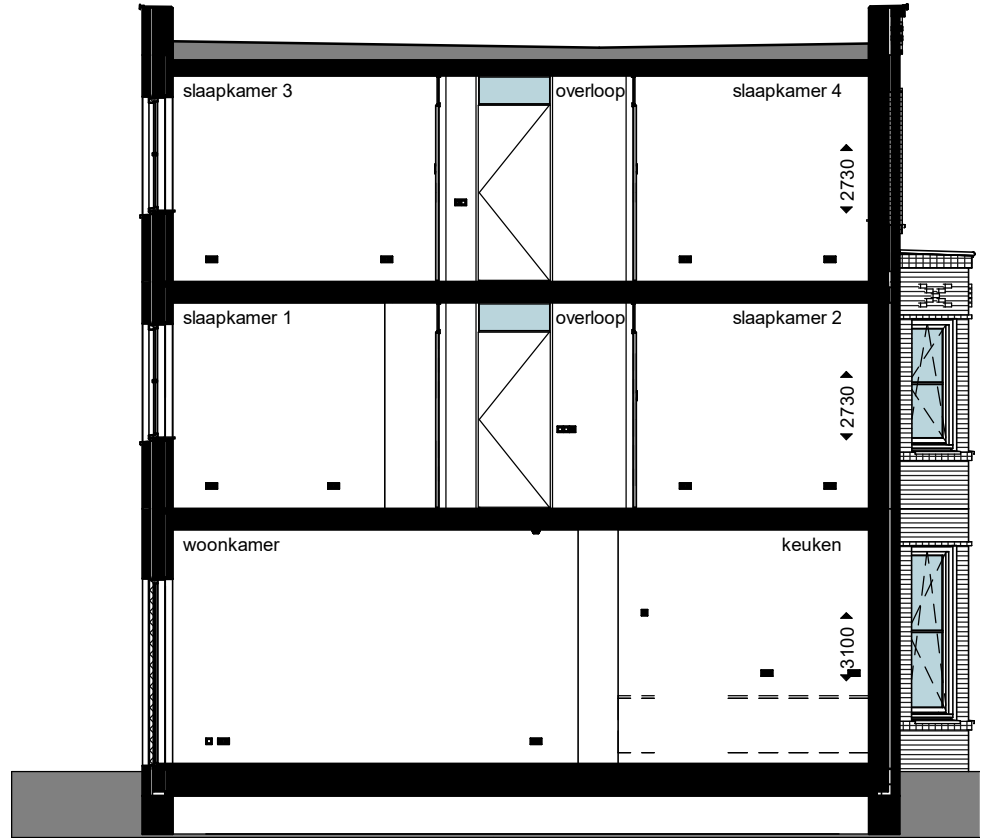
doorsnede
