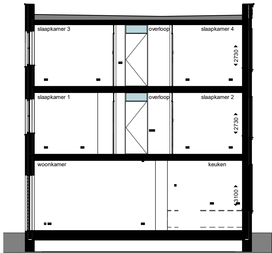
doorsnede
