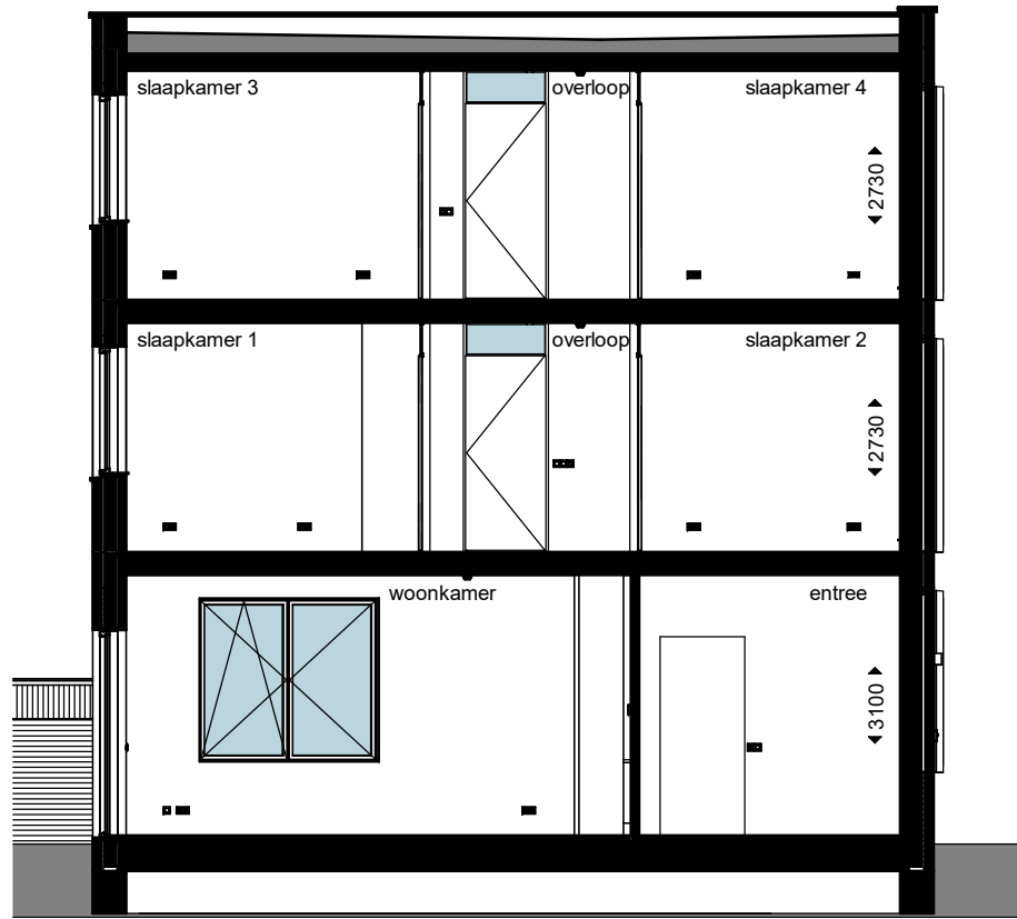
doorsnede
