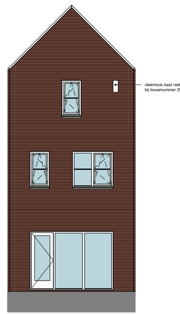
achtergevel
