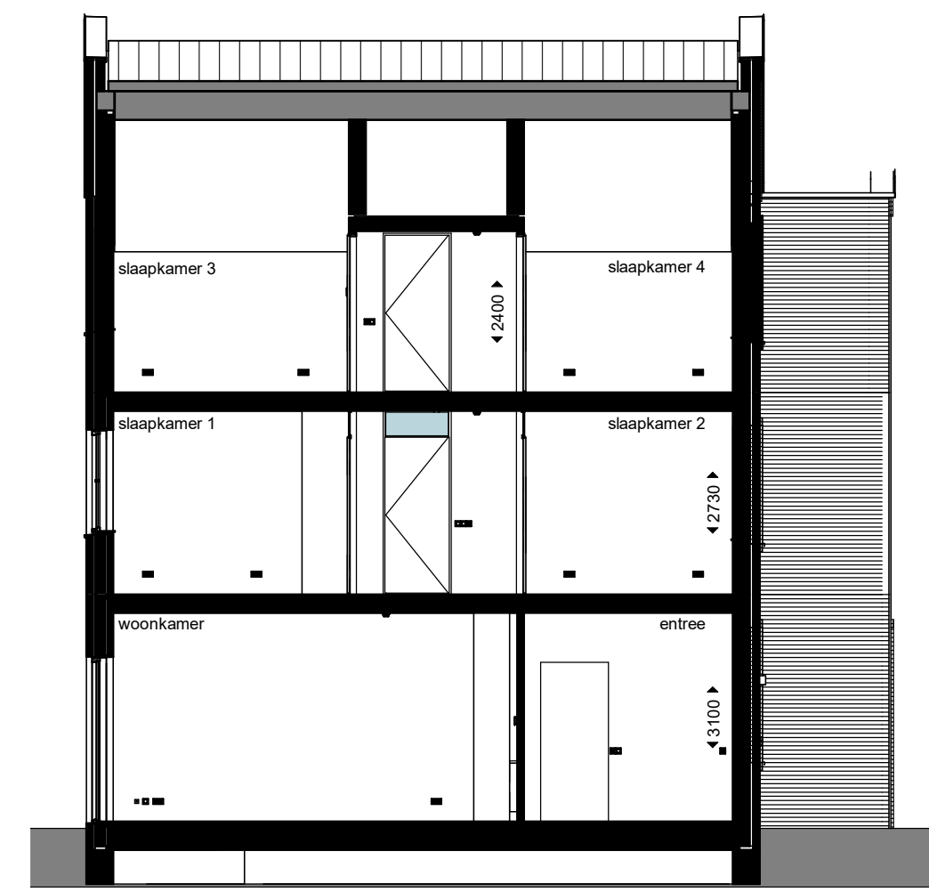
doorsnede
