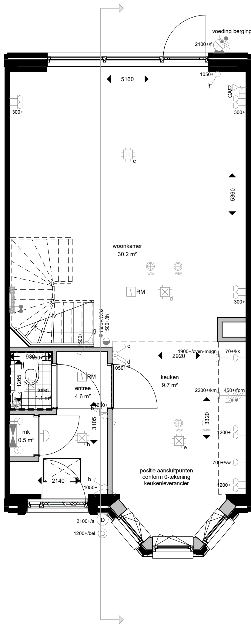
begane grond
