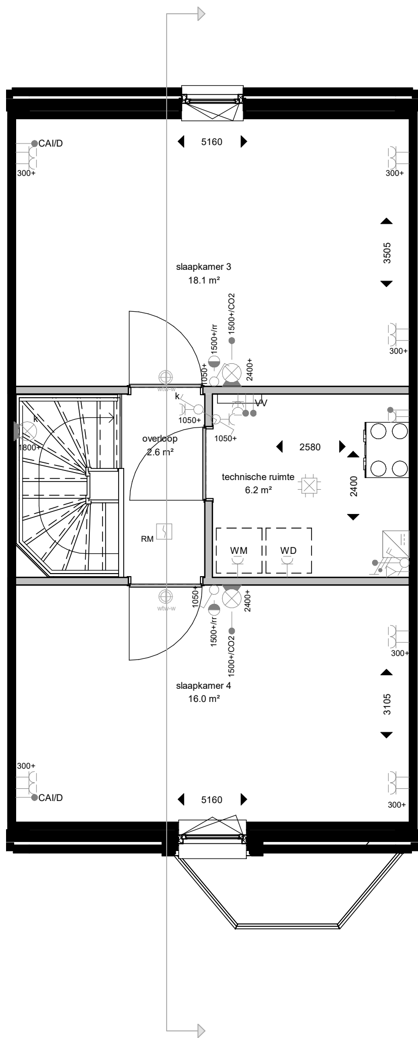
tweede verdieping
