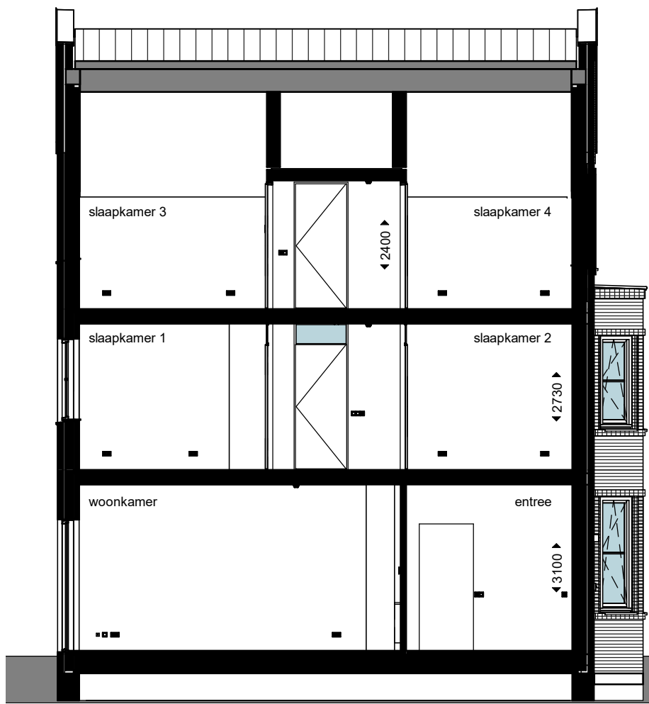
doorsnede
