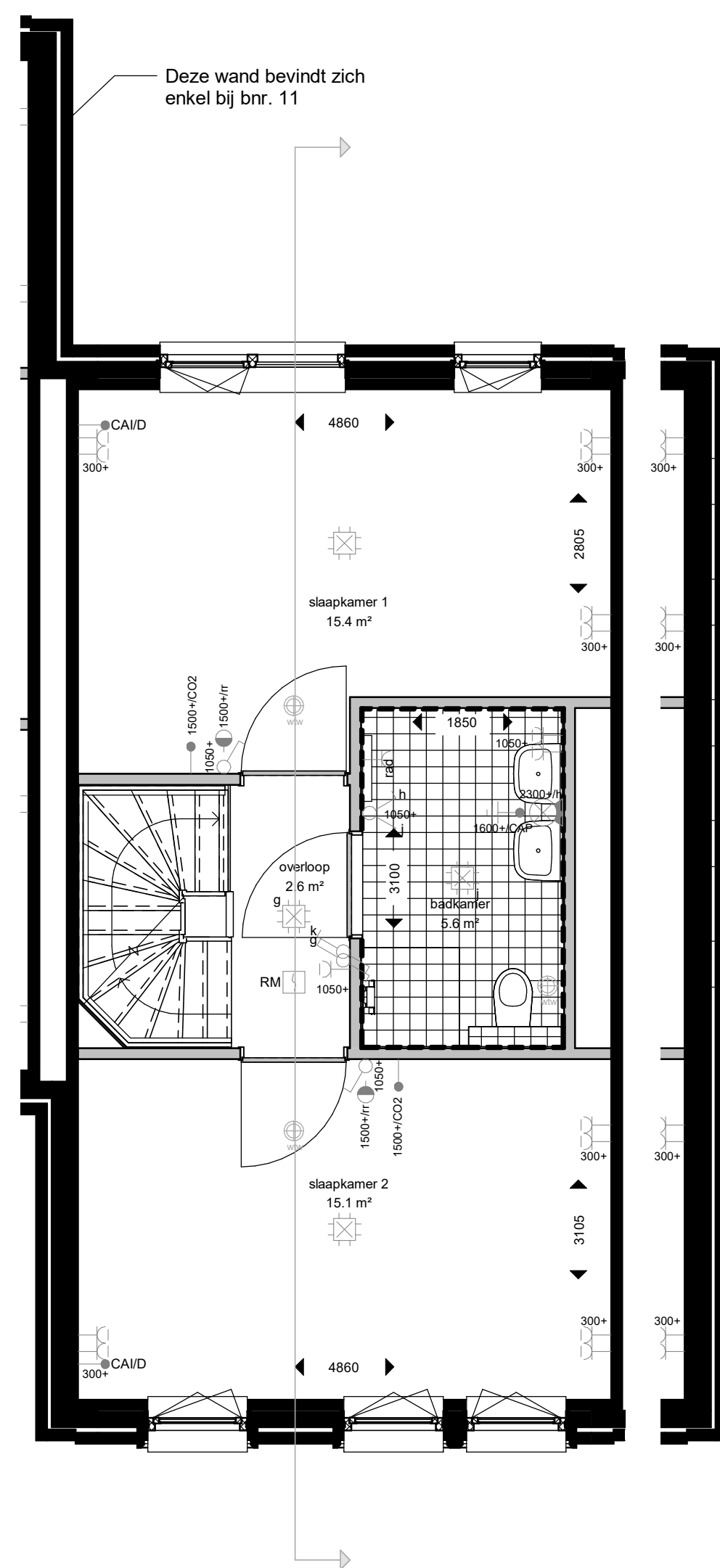
eerste verdieping
