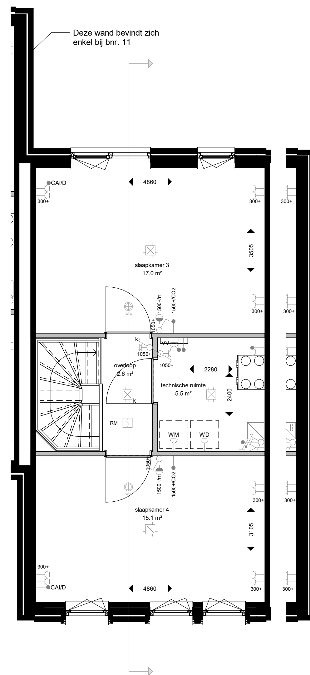
tweede verdieping
