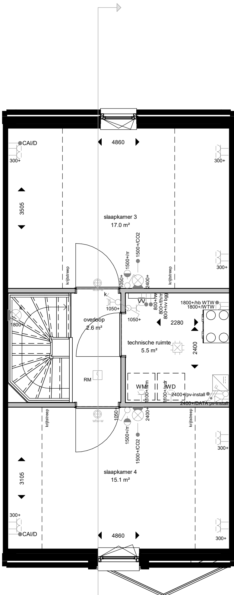
tweede verdieping
