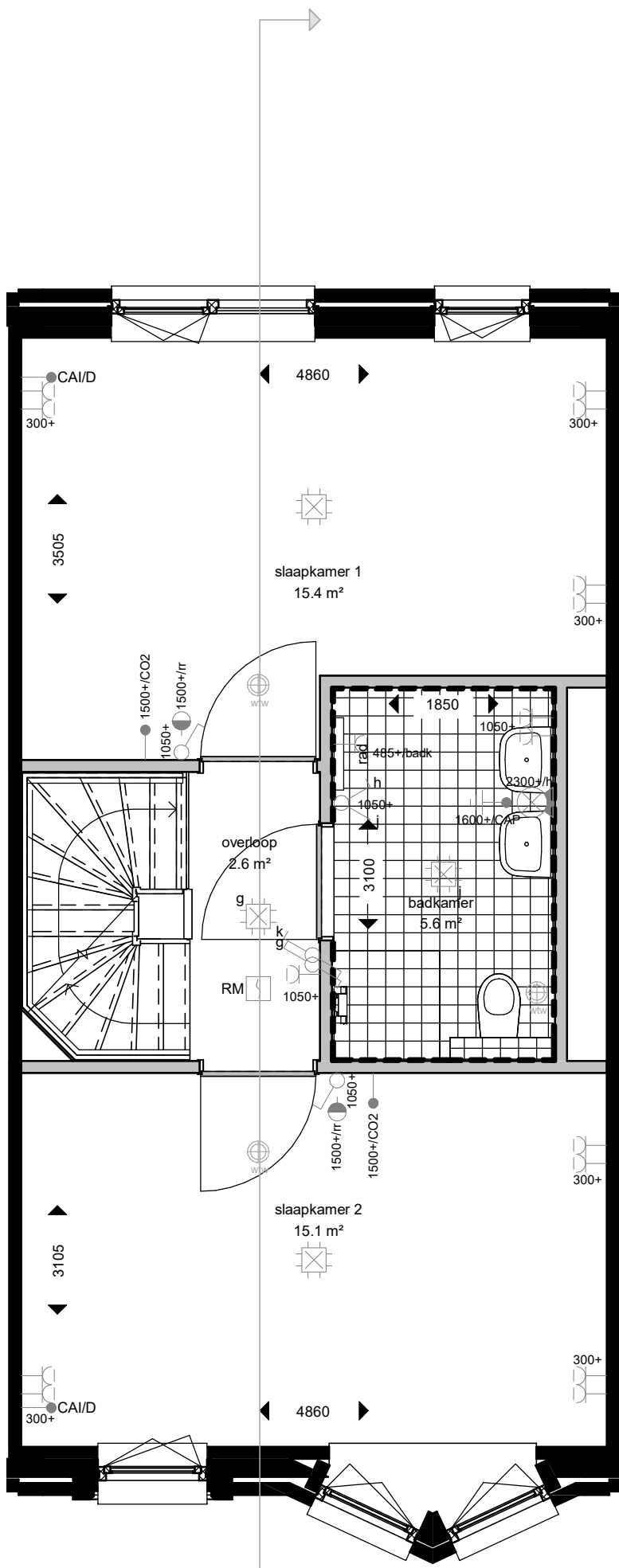
eerste verdieping
