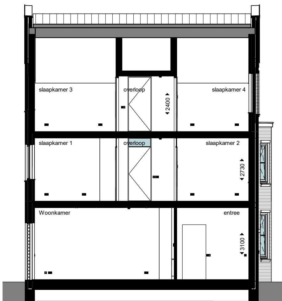
doorsnede
