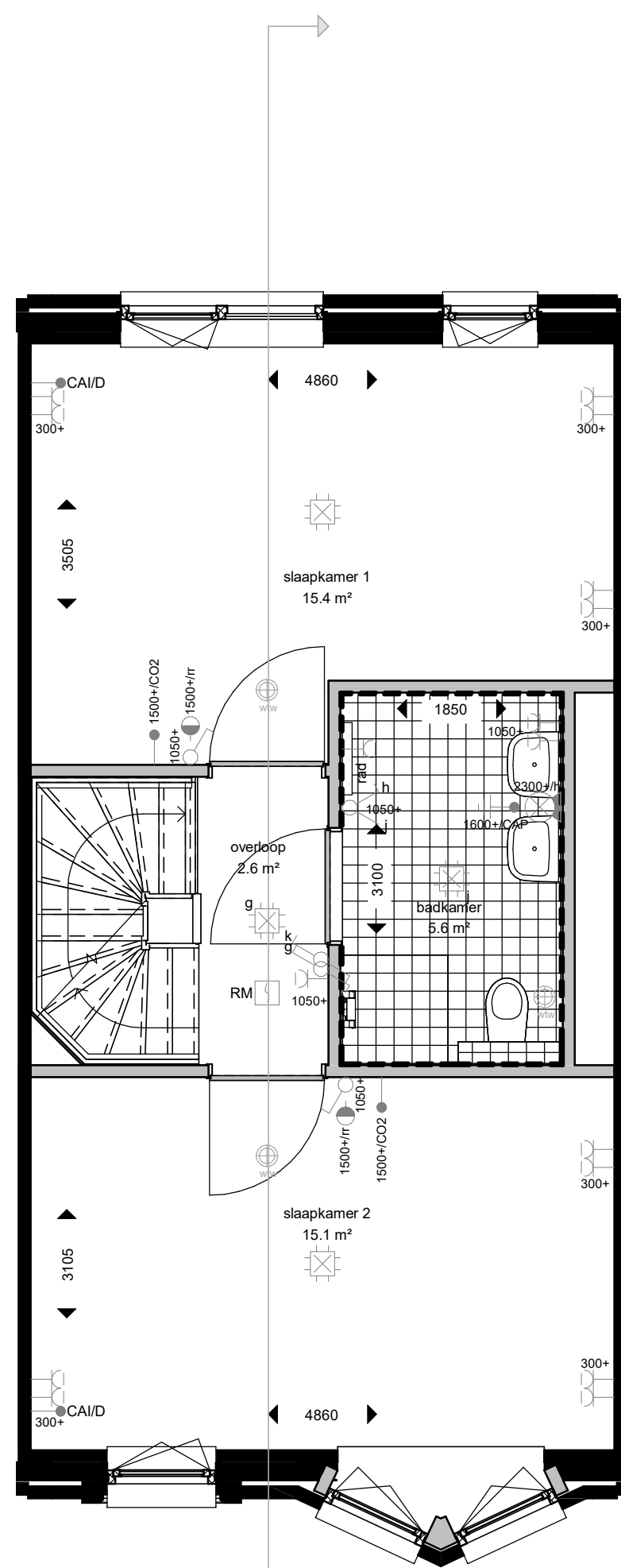
eerste verdieping
