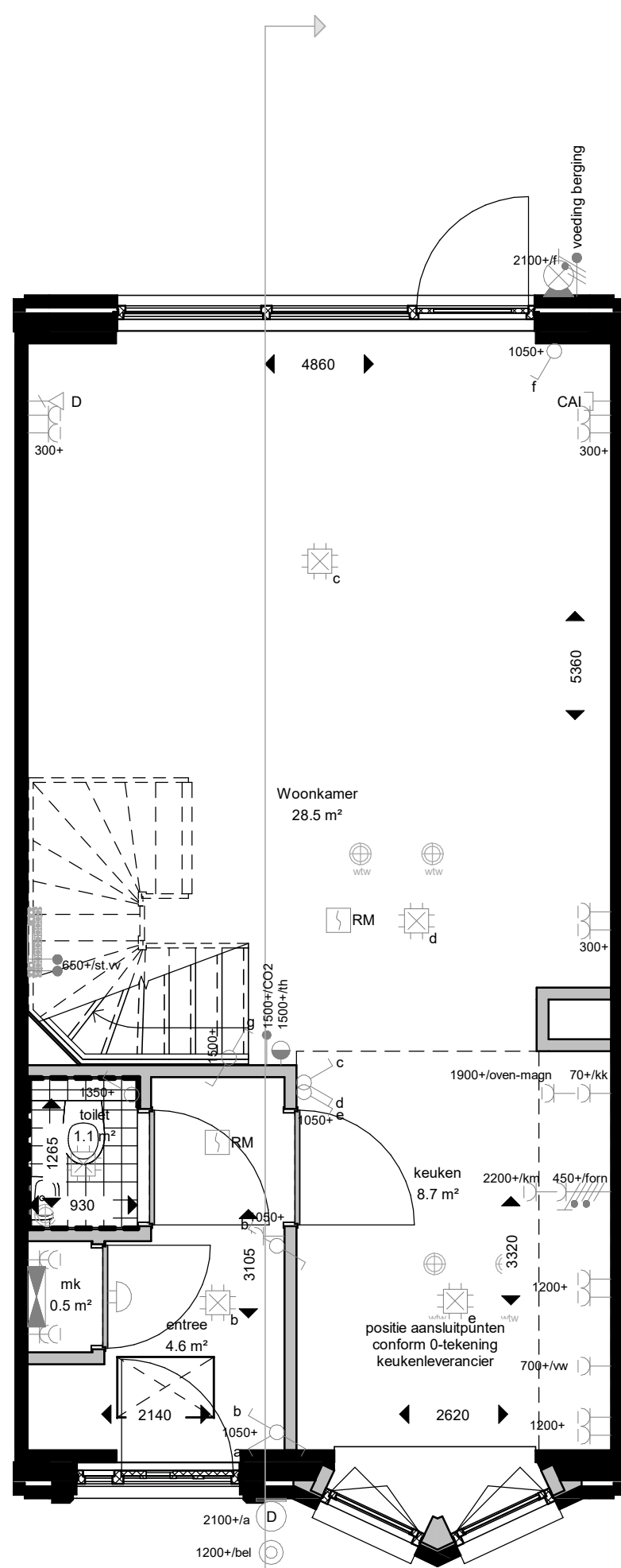
begane grond
