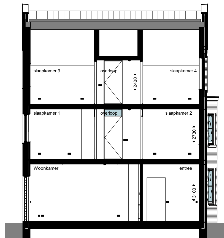
doorsnede
