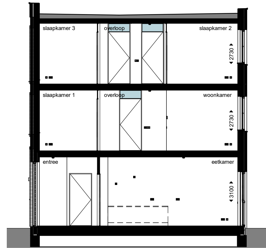
doorsnede
