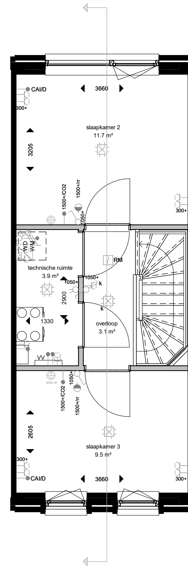
tweede verdieping
