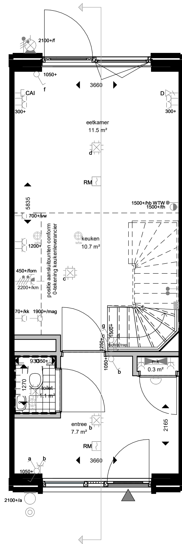
begane grond
