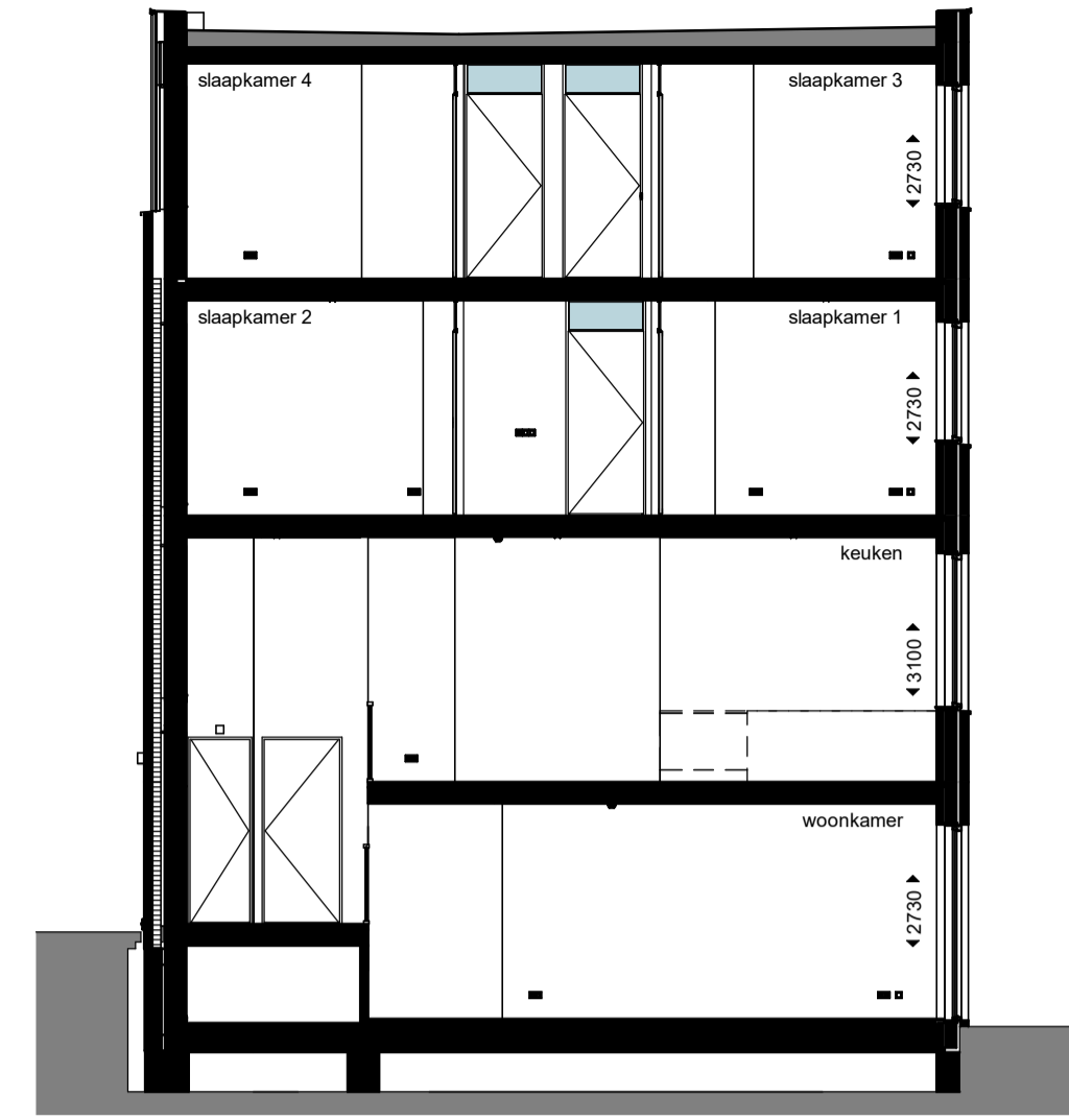
doorsnede
