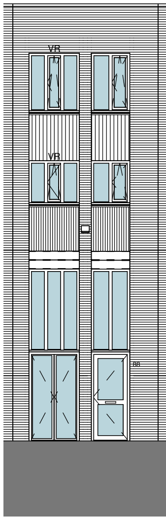
Voorgevel
