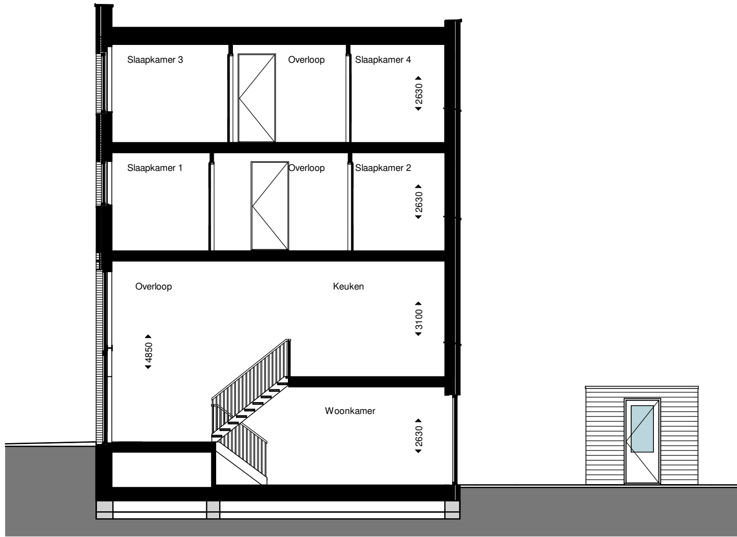
Doorsnede
