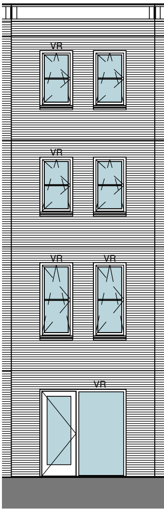
Achtergevel
